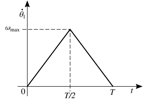
FIGURE 6 – Profil de vitesse angulaire adopté.
