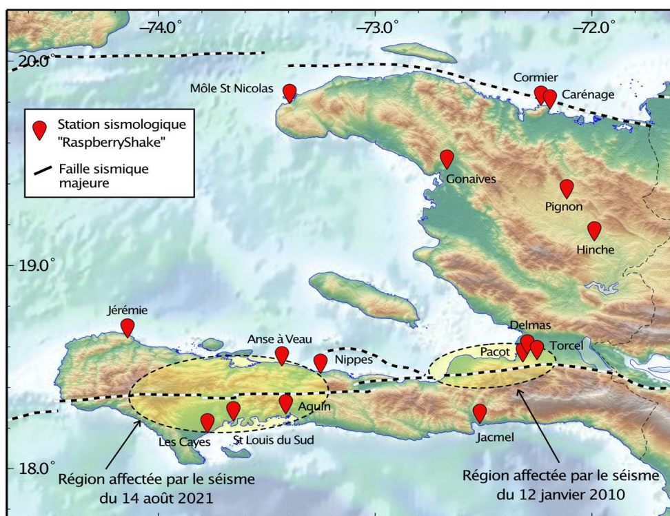
Carte des stations sismo-citoyennes RaspberryShake opérationnelles en Haïti au 24 février 2022. Les régions les plus affectées par les séismes du 12 janvier 2010 et du 14 août 2021 sont indiquées par des ellipses jaunes.
