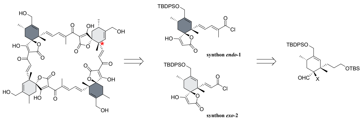
FIGURE 5 : Rétrosynthèse de la quartromicine
