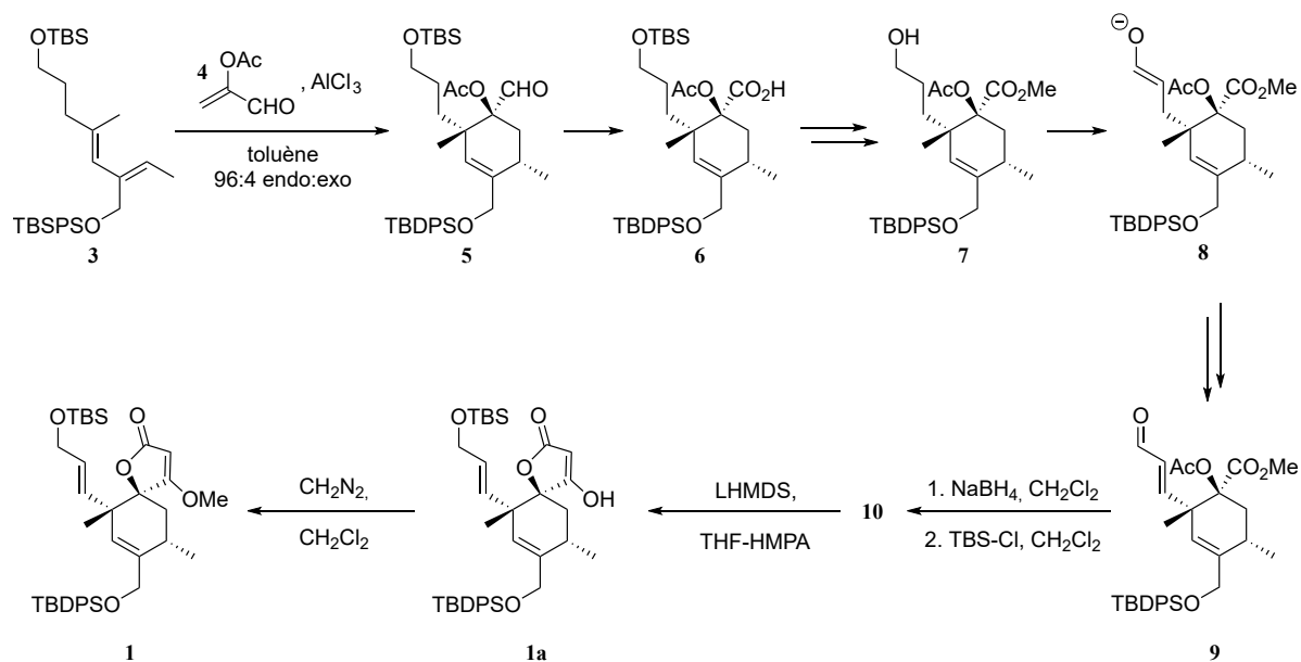
FIGURE 6 : Schéma de synthèse du composé 1
