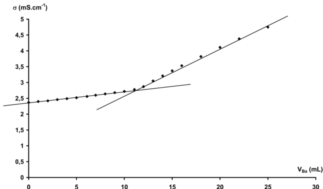
FIGURE 1 : Titrage conductimétrique de l'eau minérale par le baryum - Figure adaptée : BUP 892, Vol 101, Mars 2007, 369-379.
