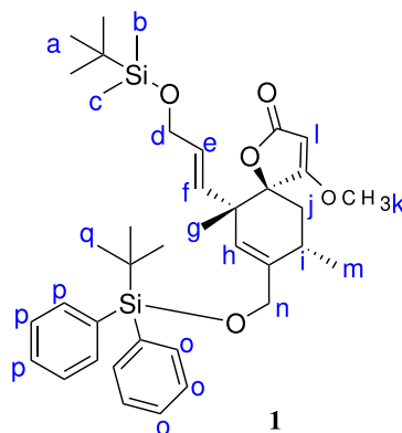
FIGURE 8 : Annotations des protons du composé 1 .
