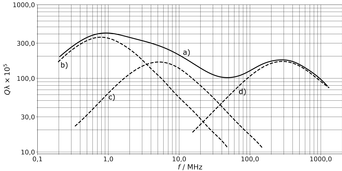
FIGURE 3 : Q\lambda en fonction de la fréquence f pour une solution aqueuse de sulfate de scandium à 0,033 \text{ mol} \cdot \text{L}^{-1} . La ligne pleine, a), représente le meilleur ajustement des données expérimentales, tandis que les lignes en pointillés, b), c) et d), montrent les contributions des effets de relaxation individuels. Figure adaptée de Bonsen et al., Ber. Bunsenges. Phys. Chem., 1978.
