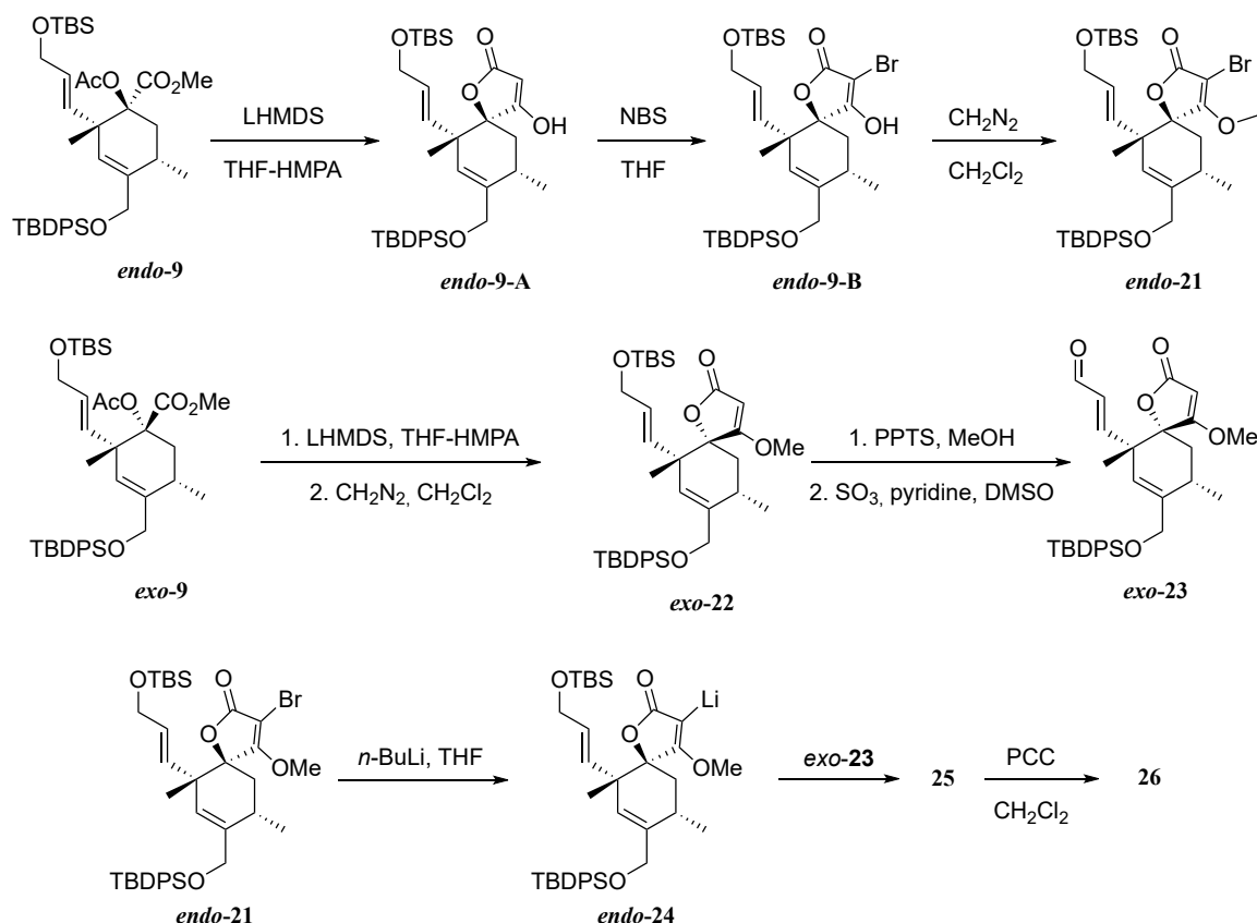
FIGURE 11 : Schéma de synthèse du composé 26
