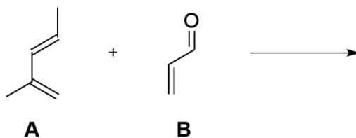
FIGURE 7 : Réaction modèle de Diels-Alder
