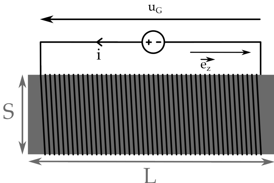
Figure 6: Dispositif expérimental pour la mise en évidence des pertes d'énergie dues aux phases irréversibles du cycle d'aimantation.
