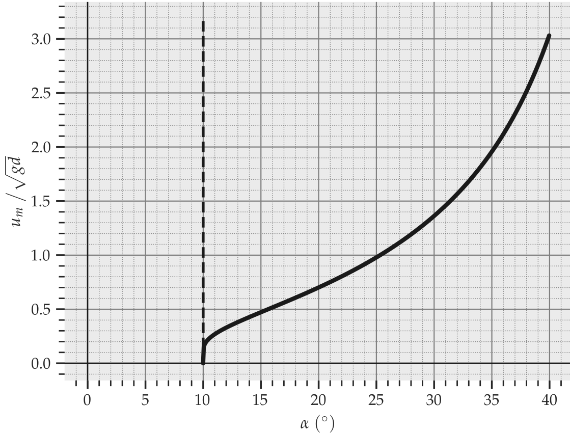
Figure 4: Vitesse d'écoulement moyenne u_m de la phase granulaire liquide, en fonction de l'angle d'inclinaison \alpha . La ligne verticale en pointillés marque l'angle critique dynamique \alpha_d .
