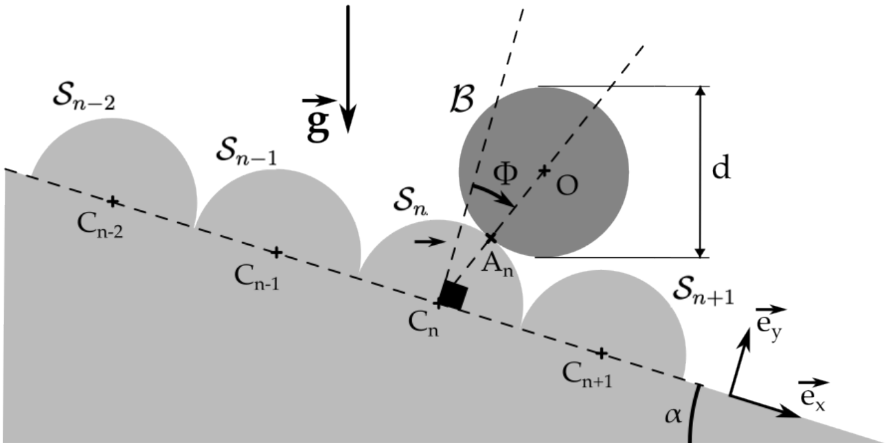
Figure 2: Modèle simplifié du milieu granulaire étudié dans la première partie.
