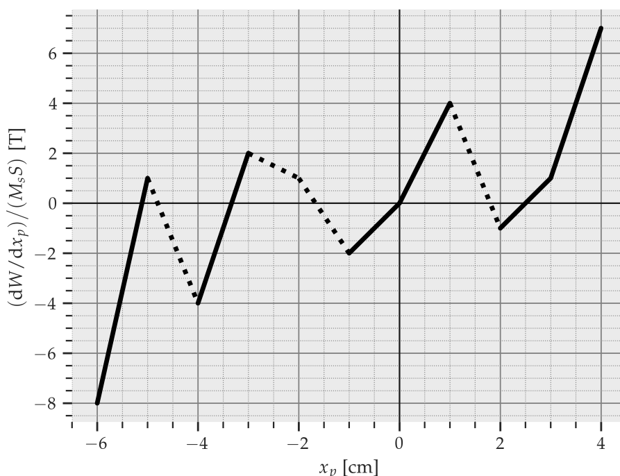
Figure 9: Dérivée par rapport à x_p de la fonction W définie à la question 63, divisée par la constante M_s S . Cette quantité a la dimension d'un champ magnétique, et est donnée en Teslas. Les branches en traits pleins sont celles où d^2W/dx_p^2 > 0 , et les branches en pointillés celles où d^2W/dx_p^2 < 0 .
